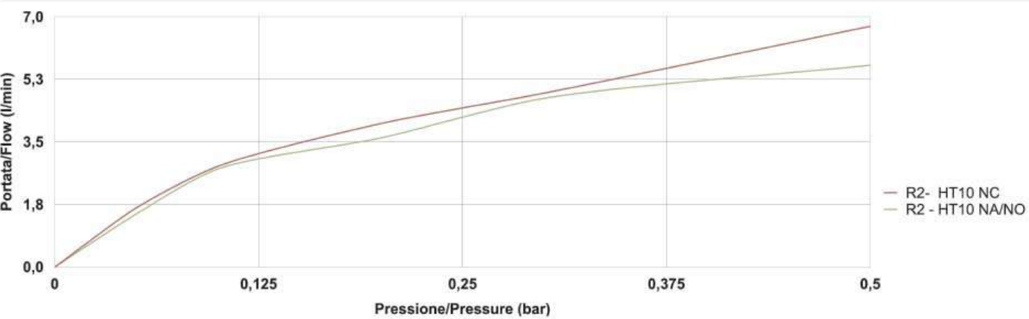
GRAFICO PORTATE SERIE R2 HT10 / FLOW RATES CHART R2 SEIRES HT10
