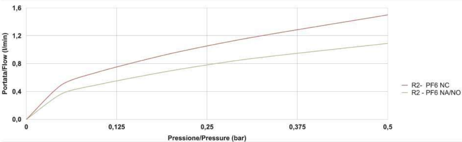
GRAFICO PORTATE SERIE R2 HTS-PF6 / FLOW RATES CHART R2 SEIRES HTS-PF6
