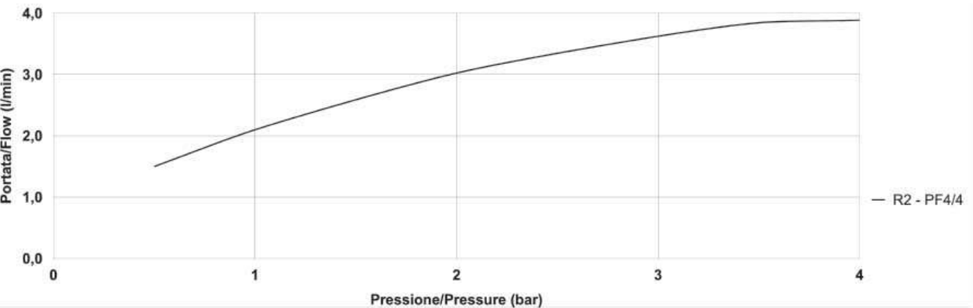
GRAFICO PORTATE SERIE R2 PF4-4 / FLOW RATES CHART R2 SEIRES PF4-4
