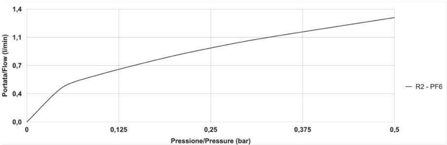
GRAFICO PORTATE SERIE R2 HTS-PF6 / FLOW RATES CHART R2 SEIRES HTS-PF6
