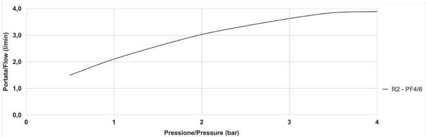
GRAFICO PORTATE SERIE R2 PF4-6 / FLOW RATES CHART R2 SEIRES PF4-6
