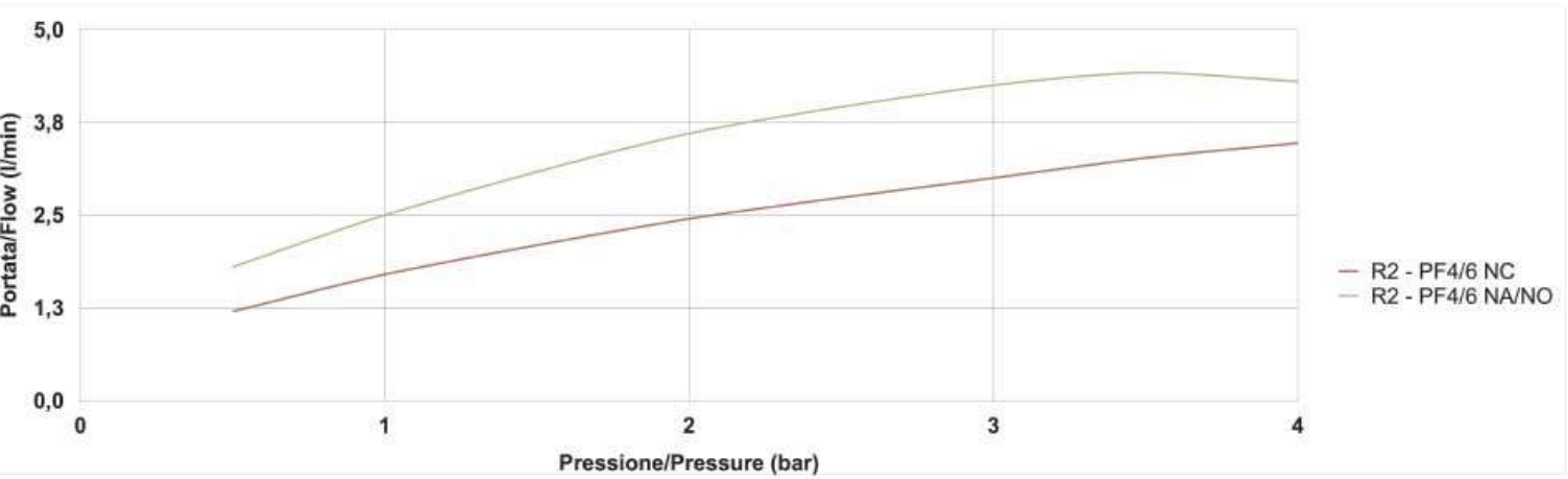
GRAFICO PORTATE SERIE R2 PF4-6 / FLOW RATES CHART R2 SEIRES PF4-6
